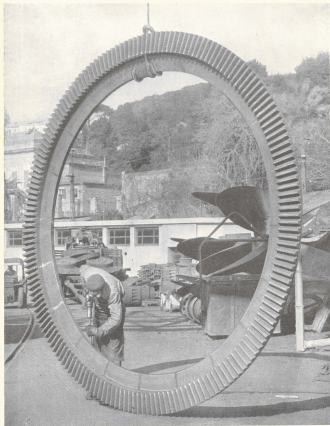
Corona dentata, del peso di 1.700 Kg. e del diametro di 1.600 mm., fatta in ghisa sferechiata partecipa fornita alla Fonderia e destinata alla completa di assemblaggio di un impianto per cemento in costruzione alla Carpenteria per il Venezuela. E' al lavoro lo scultore Anselmo Burchi.
